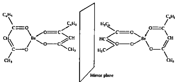
Fig. 12.3 Enantiomers of bis(benzoylacetonato)beryllium.
